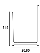
_Compensatore senza aletta/ Filler without deflector
