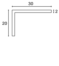
_Profilo angolare 3x2 cm/ Corner profile 3x2 cm
