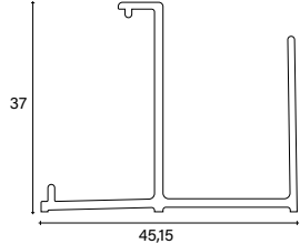
_Compensatore con aletta/ Filler with deflector
