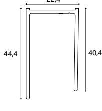
_Compensatore senza aletta/ Filler without deflector
