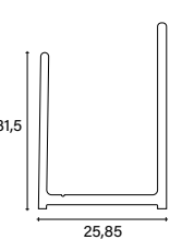
_Compensatore senza aletta/ Filler without deflector
