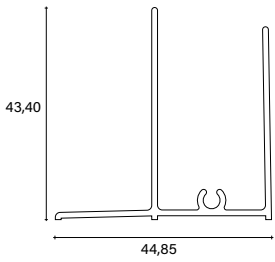
_Compensatore con aletta/ Filler with deflector
