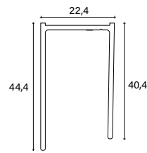
_Compensatore senza aletta/ Filler without deflector
