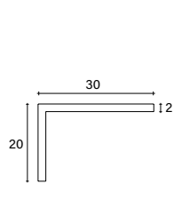
_Profilo angolare 3x2 cm/ Corner profile 3x2 cm
