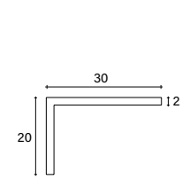
_Profilo angolare 3x2 cm/ Corner profile 3x2 cm
