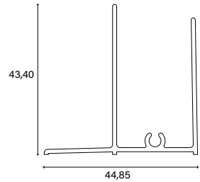
_Compensatore con aletta/ Filler with deflector
