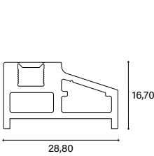
_Trafila pivot/ Pivot profile
